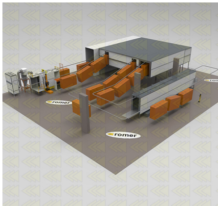
Automatische Einschienenbahn
