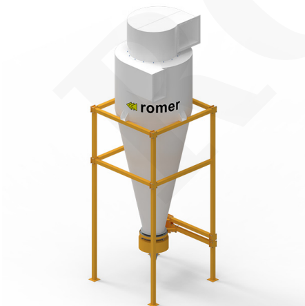
Zyklonabscheider
