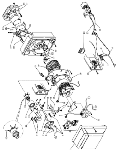
Teile für den RIELLO-Gasbrenner
